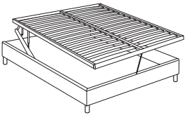
LEVITEC dispositivo di sollevamento per letto matrim. 165 LEVITEC lifting device for the 165 king-size bed
