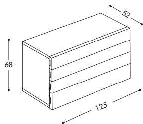
VASTO COMÒ 4 cassetti - 4 drawers
