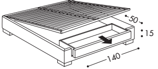
PEDIERA CON CASSETTO per letto matrim. 165 FOOT BOARD WITH DRAWER for the 165 king-size bed
