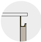
Frontali con maniglia integrata Fronts with integrated handle
