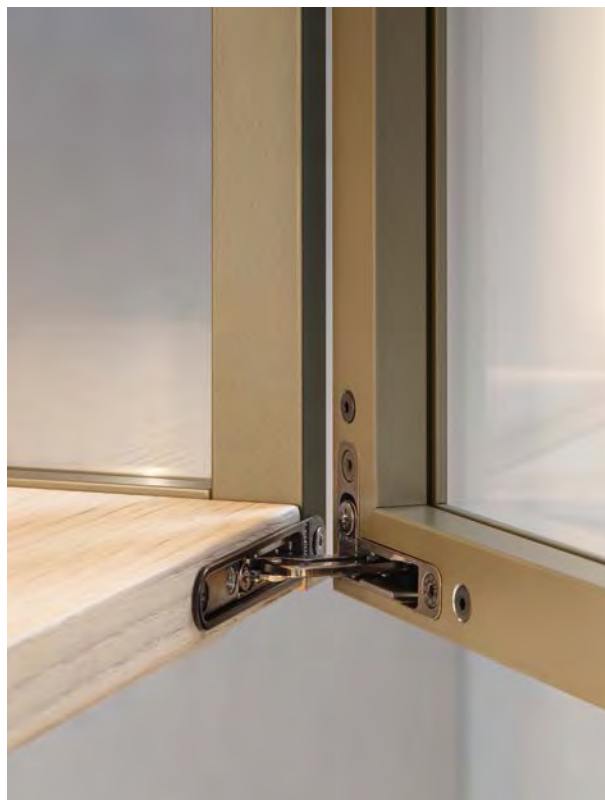
guscio per cerniera, brevetto internazionale hinge shell, international patent
