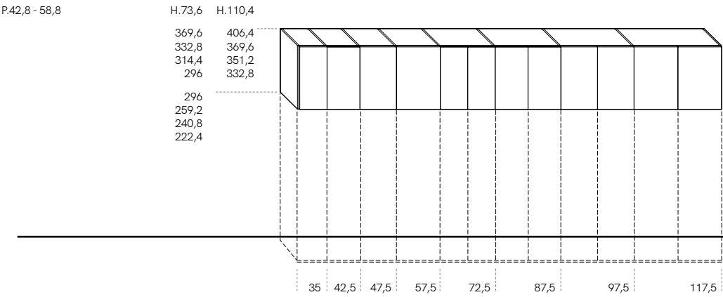
Moduli sovrapponibili Overhead modules
